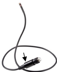
Fig. 39: Sonda Wöhler VE 400, Ø 5,5mm, tasto per la commutazione da vista 0° a vista 90°.
